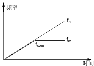
图 6-9 开环主辅给定运算 5
