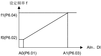
图 6-20 设定频率特性曲线（正作用）
