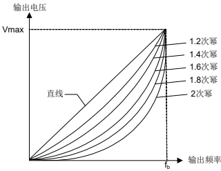
图 6-10 V/F 曲线
