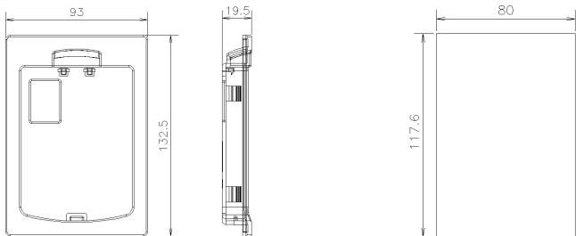
托板（V6-DP05）
