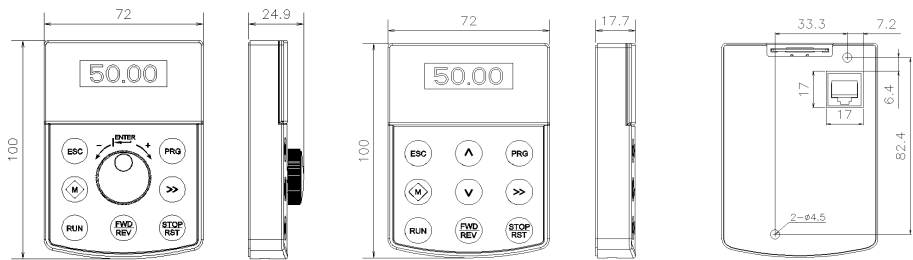
飞梭型操作面板（V6-DP01）
