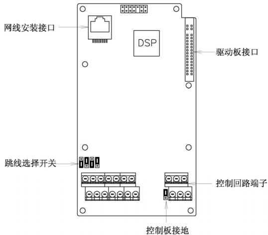
图 3-8 E5-H / E5-P 控制板示意图
