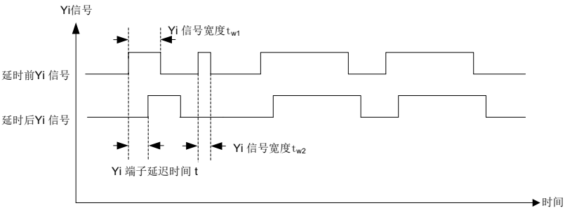
图 6-27 输出端子 Yi 延时
