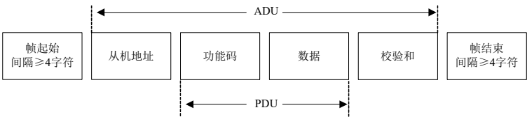
附图2 协议格式
