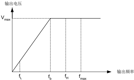
图 6-2 特性参数定义
