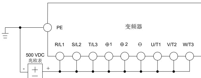
图8-2 E5-H-4T18.5GX~E5-H-4T500GX主回路绝缘测试 E5-P-4T22X~E5-P-4T560X主回路绝缘测试 E5-A-4T22X~E5-A-4T450X主回路绝缘测试
