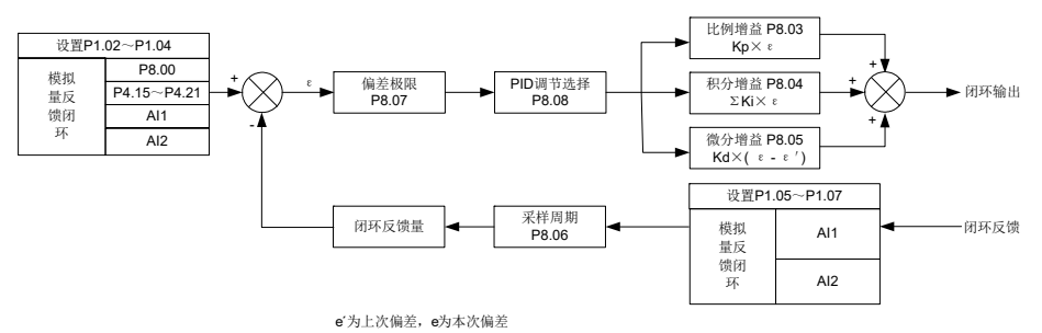
图 6-30 PID 原理框图
