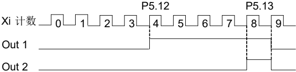
图 6-17 预置和到达计数值给定示意图
