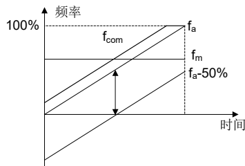
图 6-7 开环主辅给定运算 3
