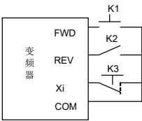
图 6-16 三线式运行模式 2
