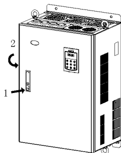
图 2-11 打开门板
