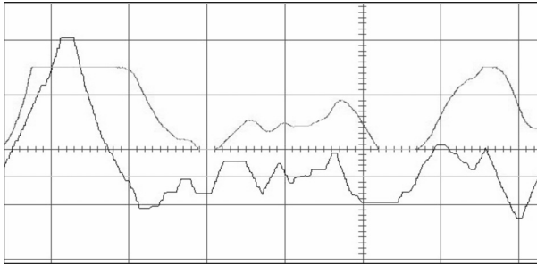
P8.08=00,P8.09=1: 到达上下限禁止积分,反作用
