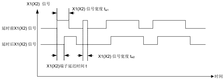
图 6-12X1/X2 端子延时
