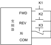
图 6-15 三线式运行模式 1
