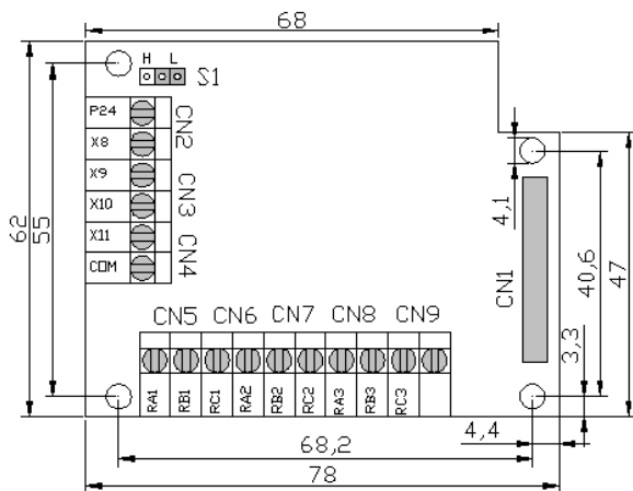
图 2-2 EX-DT01 外形尺寸 (mm)
