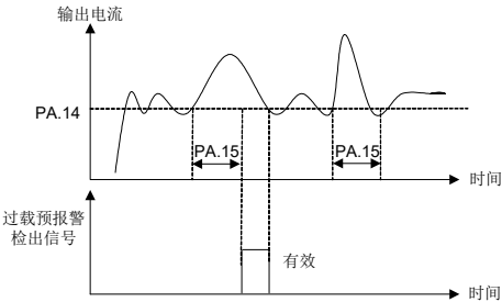
图 6-33 过载预警检出信号
