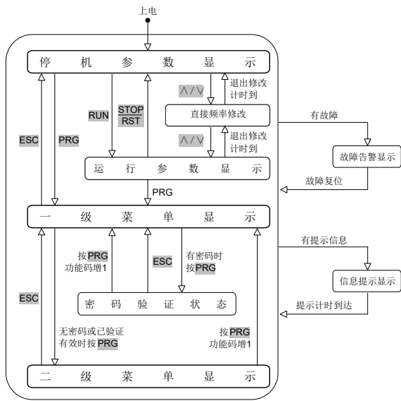
图 4-5 显示状态及操作流程
