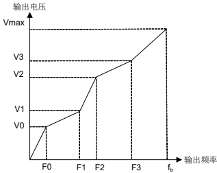
图 6-11 多段 V/F 曲线
