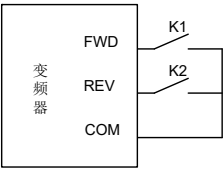
图 6-13 两线式运行模式 1
