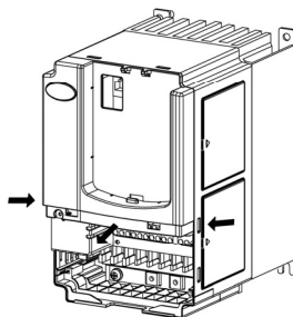
图 2-6 上盖板的拆卸
