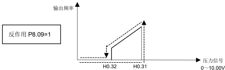
压力控制休眠启停（反作用）
