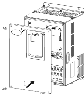
图 2-10 安装盖板
