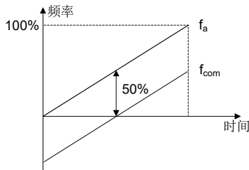
图 6-6 开环主辅给定运算 2
