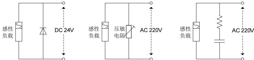
图 3-5 感性负载浪涌抑制器的应用
