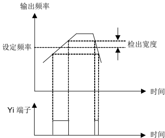
图 6-28 频率到达信号 FAR
