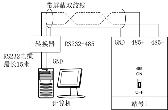
附图 3 一台变频器与计算机的连接
