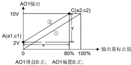
图 6-24 AO1 特性曲线 kx+b
