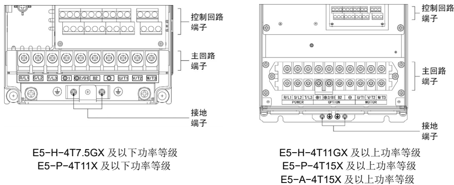
图 3-2 产品端子配置情况
