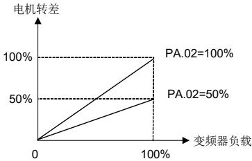
图 6-32 转差补偿增益
