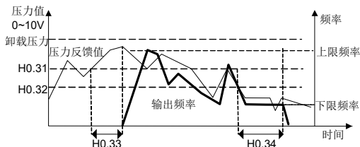
图 6-37 压力控制休眠启停保持时间
