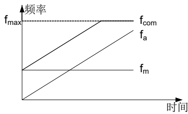
图 6-4 开环主辅给定运算 0
