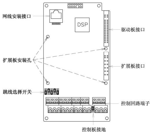
图 3-9 E5-A 以及 E5-H-34/ E5-H-63、E5-P-34/ E5-P-63 控制板示意图
