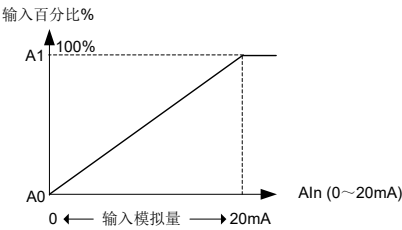
图 6-19 输入模拟量（电流）对应百分比
