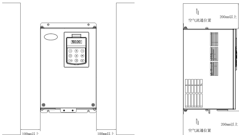
图 2-2 E5-H-4T11GX / E5-P-4T15X / E5-A-4T15X 及以上功率等级的安装方向和空间
