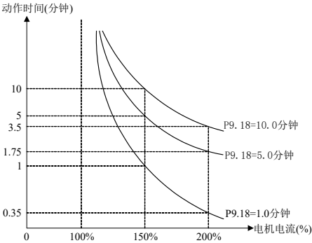
图 6-31 电机过载保护特性曲线（恒转矩）
