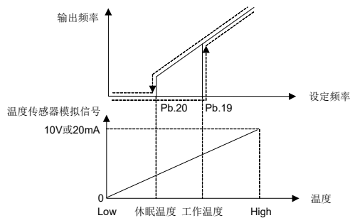
图 6-35 零频运行上下界
