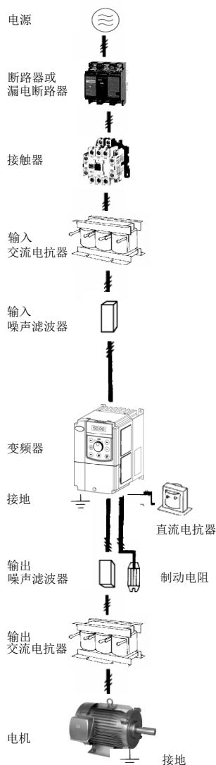
图 3-1 产品与外围器件的连接图
