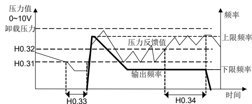
图 6-36 压力控制休眠启停保持时间
