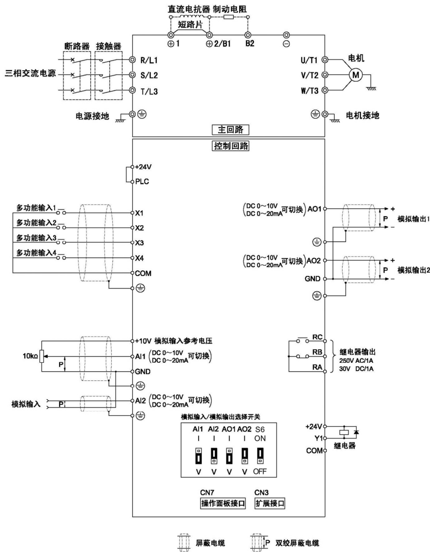
图 3-6 端子配线图（以 E5-H-4T5.5GX 型举例）
