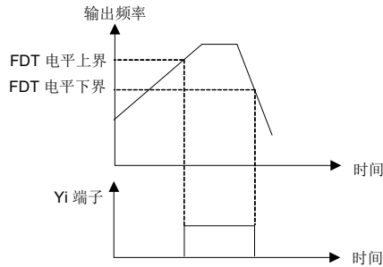
图 6-29 频率水平检测信号 FDT
