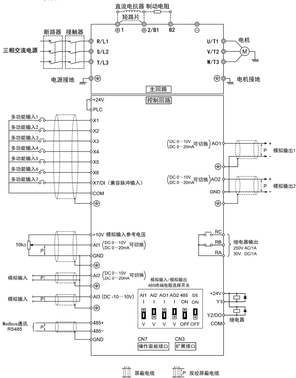
图 3-7 端子配线图 (以 E5-H-4T5.5GX-34 型举例)
