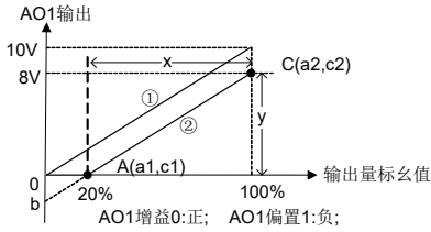
图 6-25 AO1 特性曲线 kx+b
