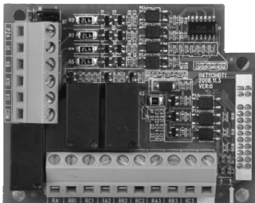
图 2-1 (EX-DT01 外观)
