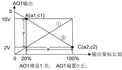
图 6-26 AO1 特性曲线 kx+b
