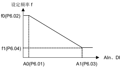
图 6-21 设定频率特性曲线（反作用）
