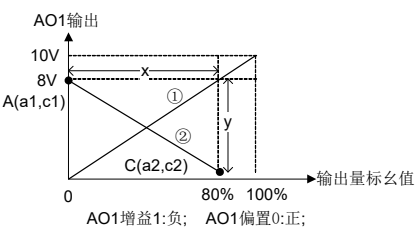
图 6-27 AO1 特性曲线 kx+b
