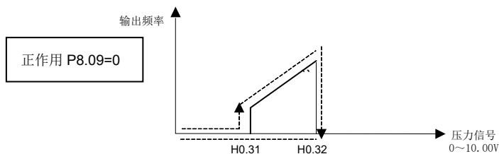
压力控制休眠启停（正作用）
