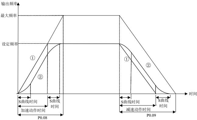
图 6-1 加减速时间及 S 段曲线
