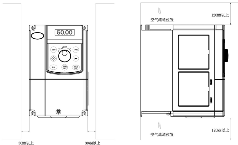
图 2-1 E5-H-4T7.5GX / E5-P-4T11X 及以下功率等级的安装方向和空间
