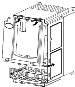
图 2-7 上盖板的安装
