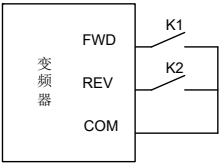
图 6-14 两线式运行模式 2
