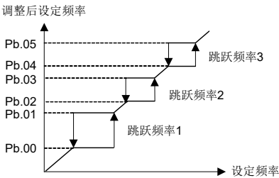
图 6-34 跳跃频率上下限
