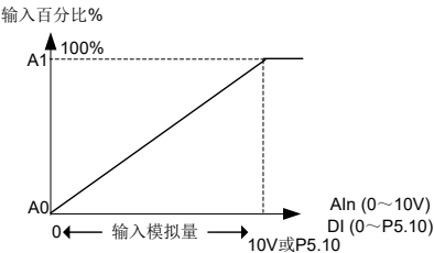
图 6-18 输入模拟量（电压/频率）对应百分比
