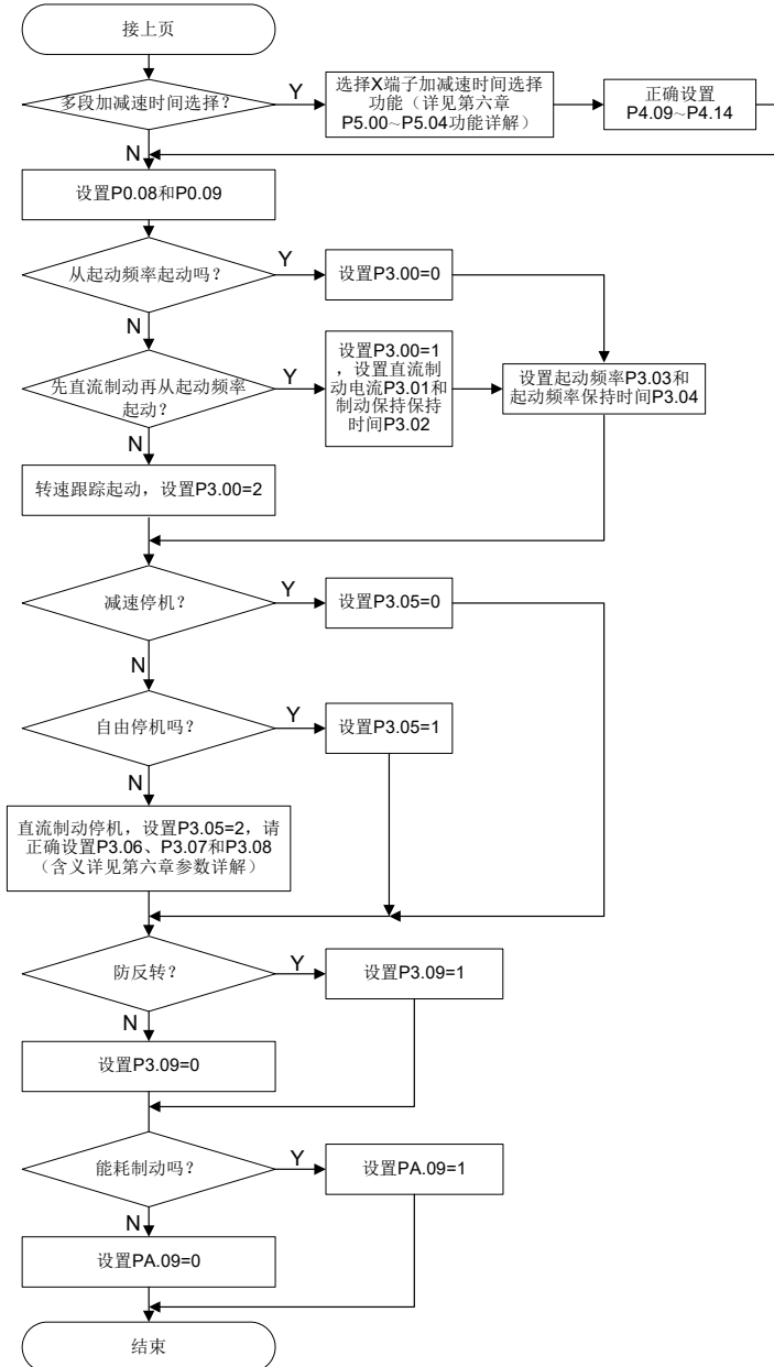
过程闭环的设置流程（续）
