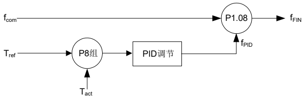
图 6-10 开环和闭环复合运行给定
