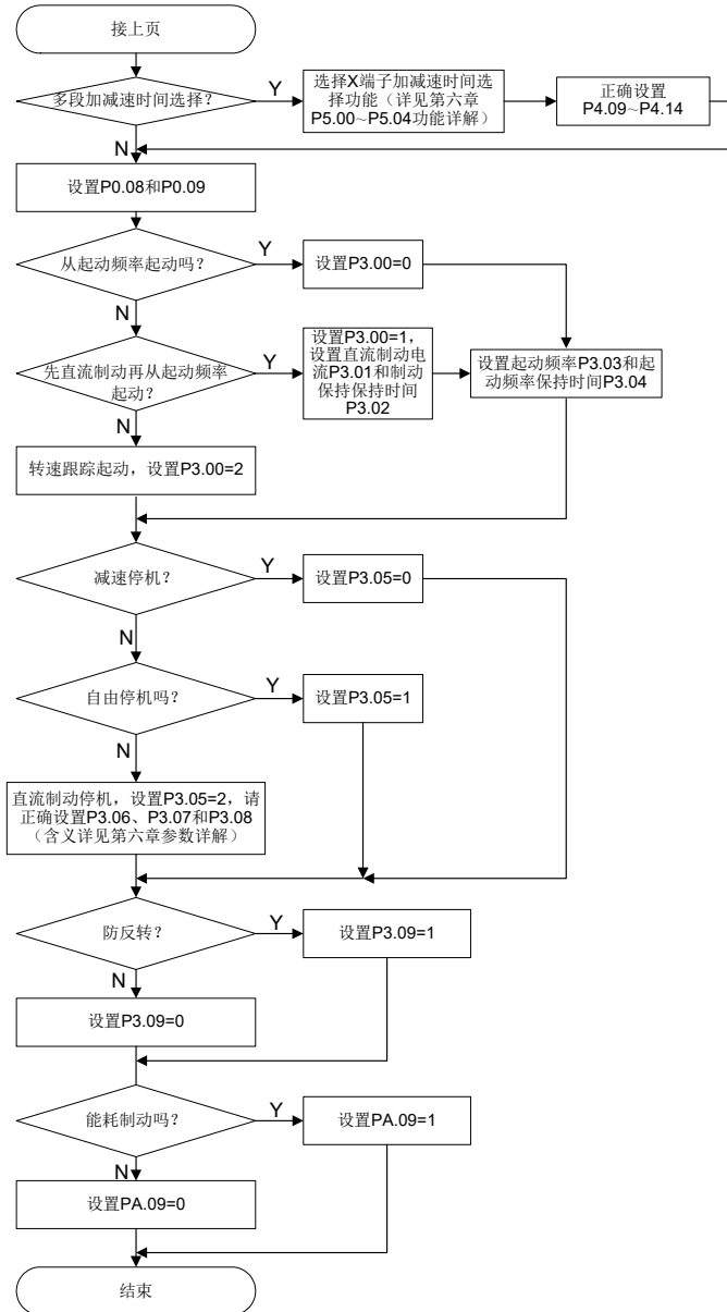
过程开环的设置流程（续）
