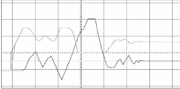
P8.08=00,P8.09=0: 到达上下限频率禁止积分,正作用
